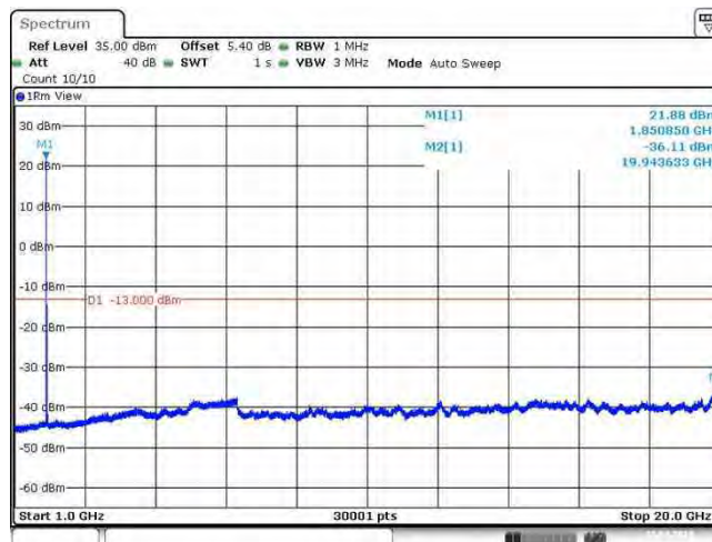
Band2_20MHz_QPSK_18700_1RB#0
