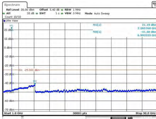
Band41_20MHz_QPSK_40640_1RB#0
