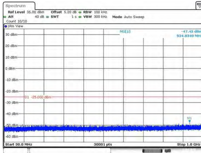
Band41_20MHz_QPSK_40640_1RB#0
