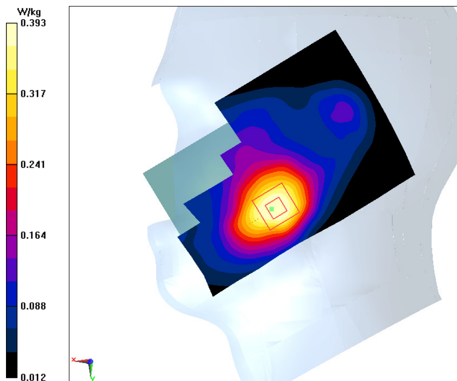
Fig.7 1700MHz
