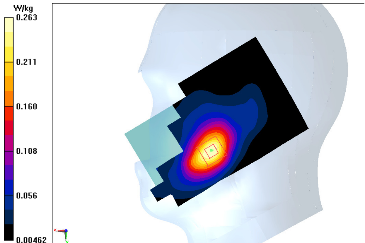
Fig.11 LTE Band2
