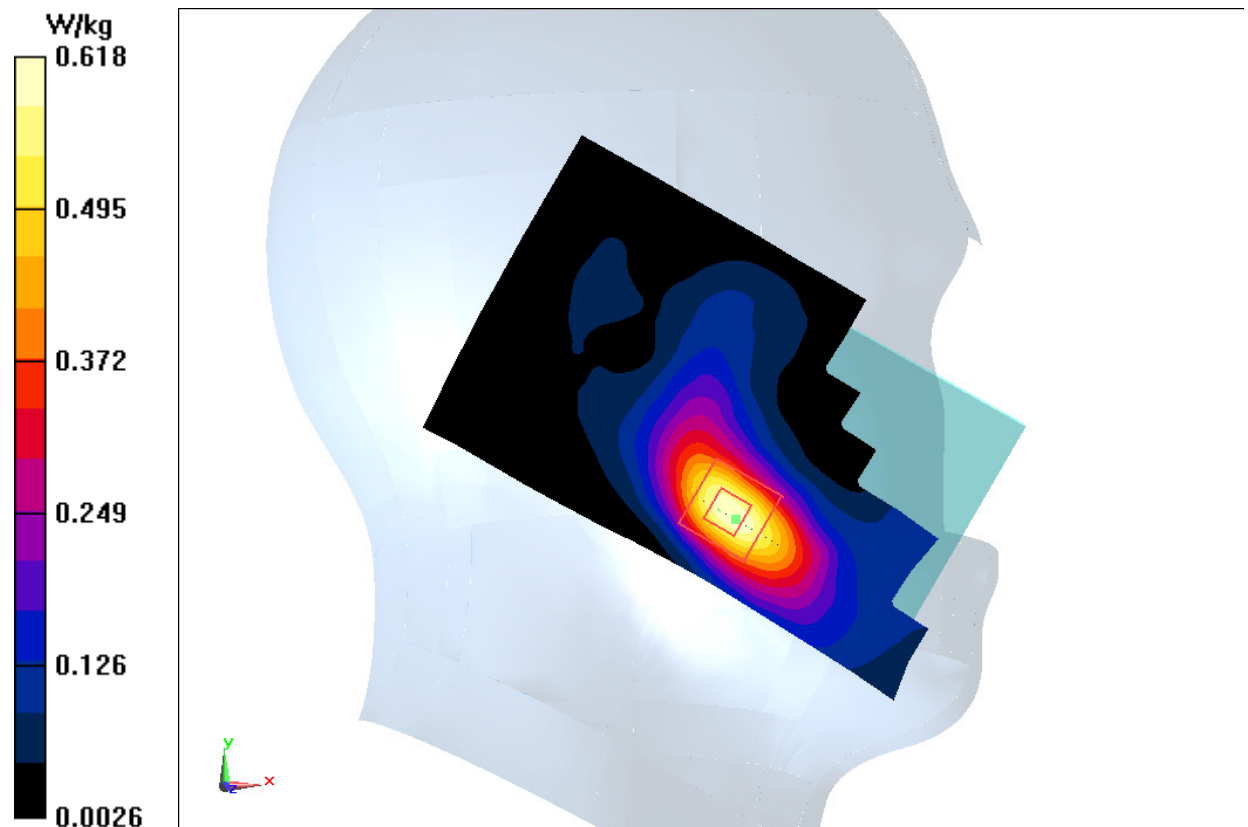
Fig.17 LTE Band7
