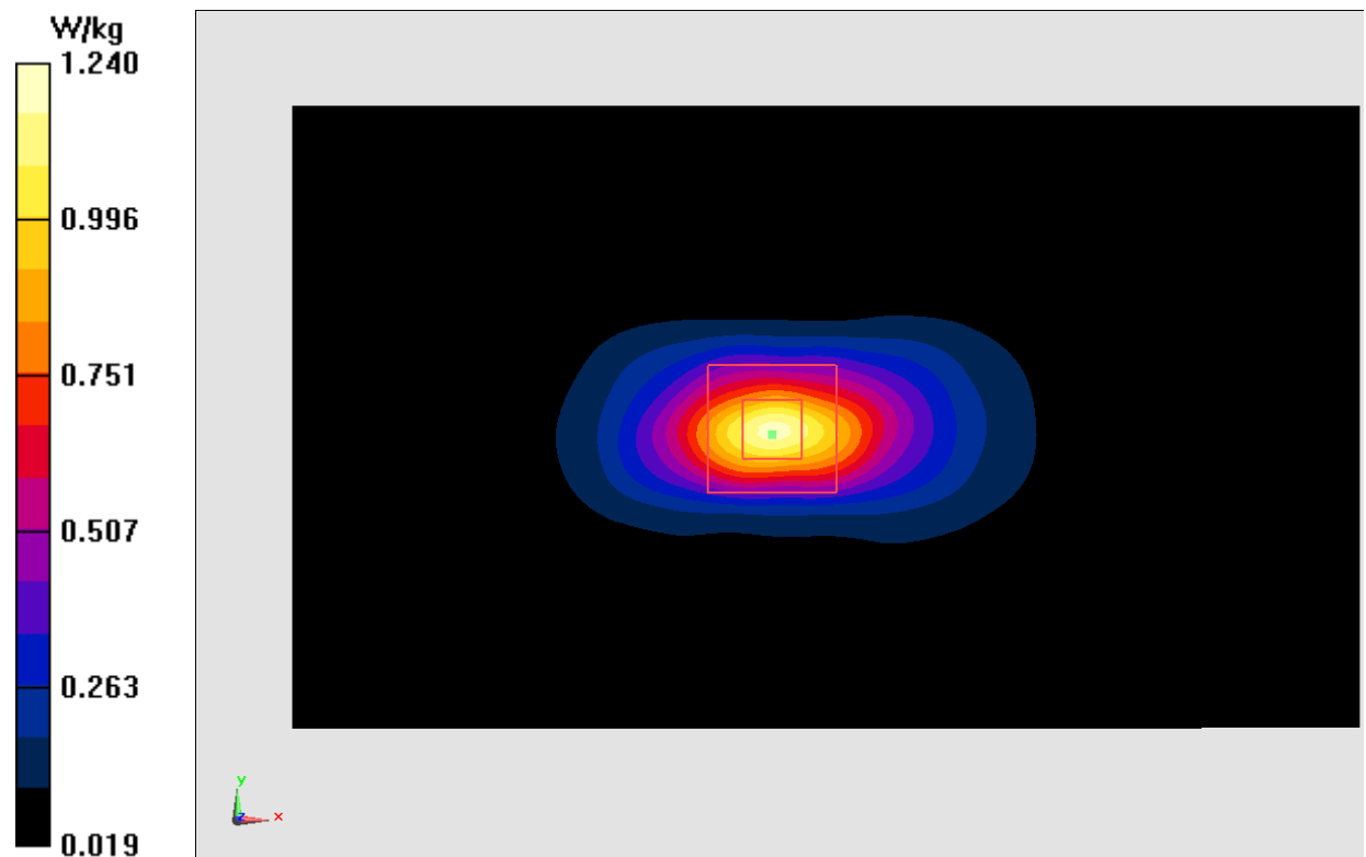
Fig.12 LTE Band2
