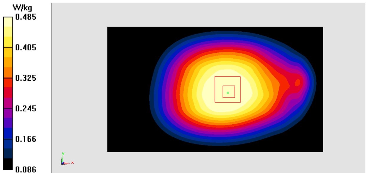
Fig.16 LTE Band5
