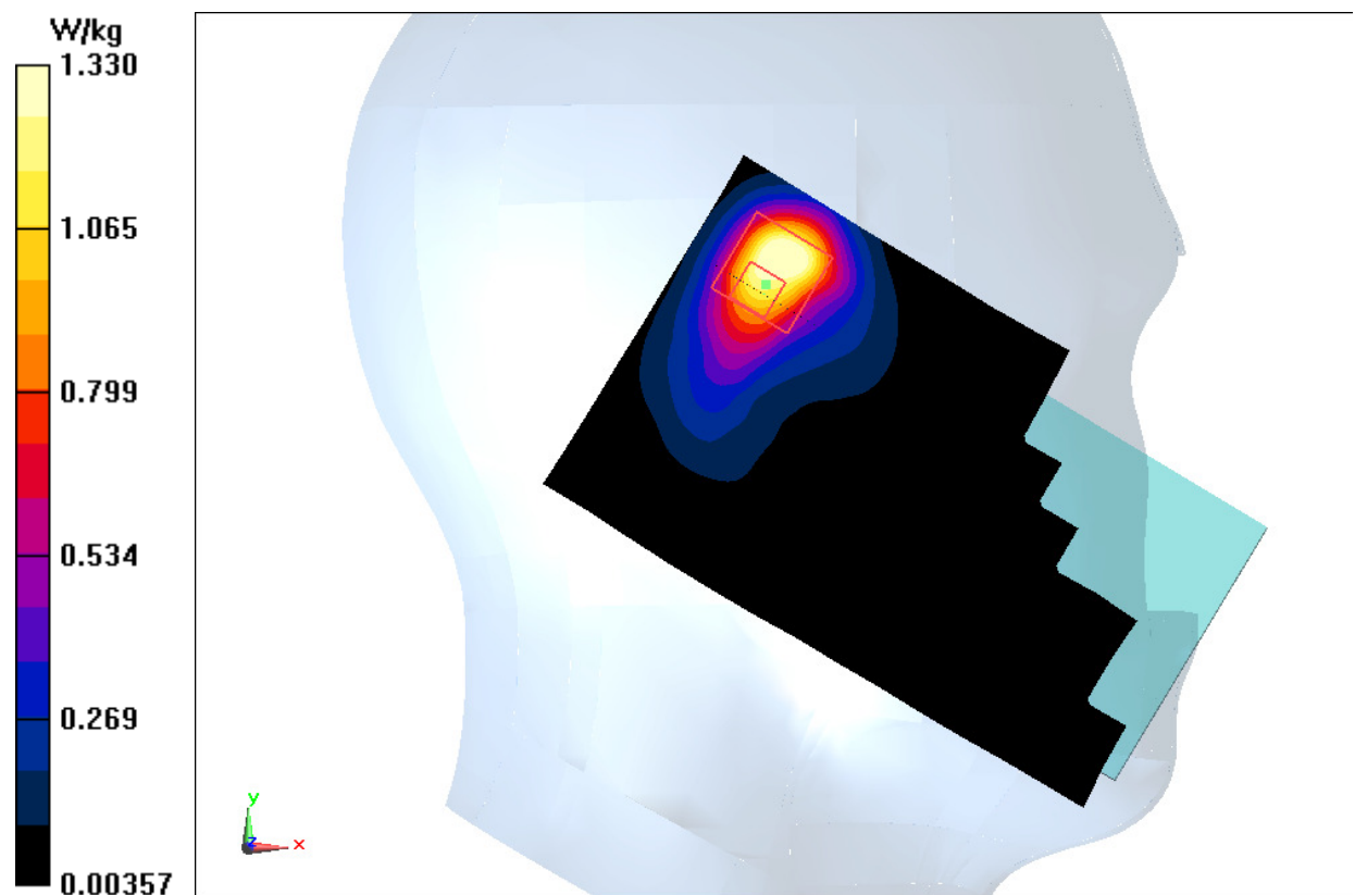
Fig.19 2450 MHz
