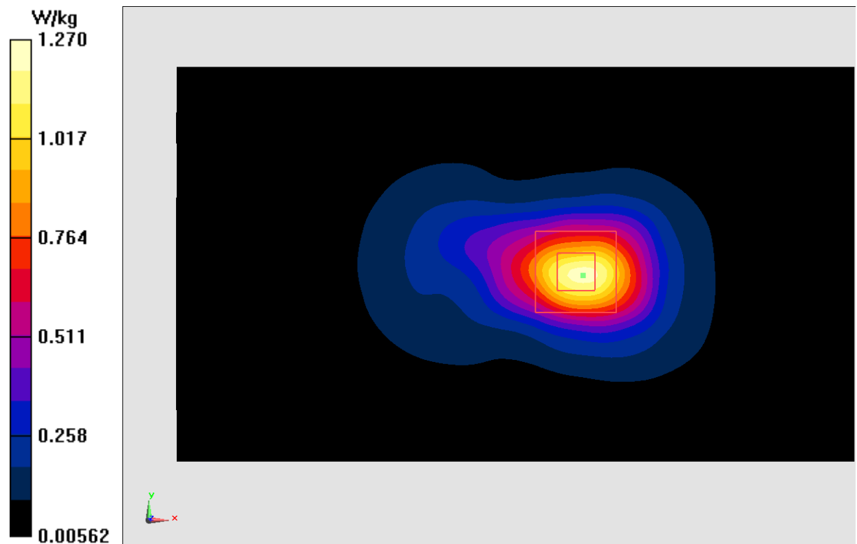
Fig.18 LTE Band7
