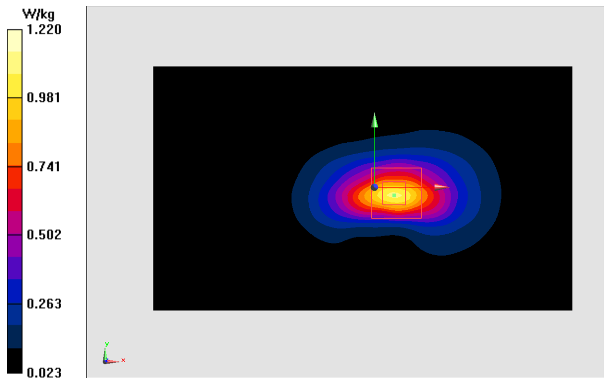
Fig.14 LTE Band4
