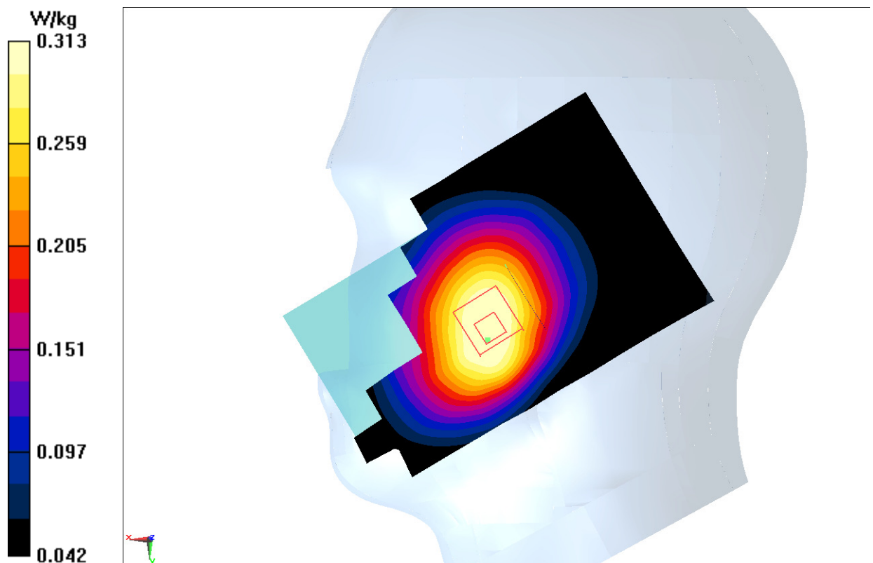
Fig.15 LTE Band5
