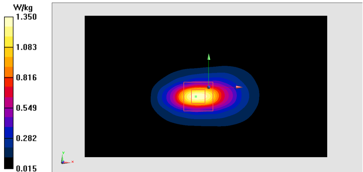
Fig.10 WCDMA1900
