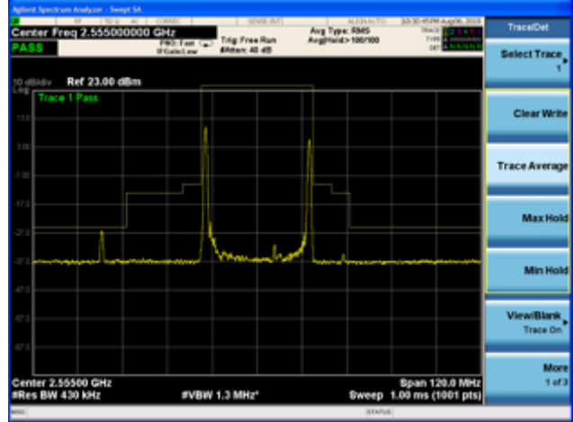
CA-7C QPSK 20MHz+10MHz CH-High, 100%RB
