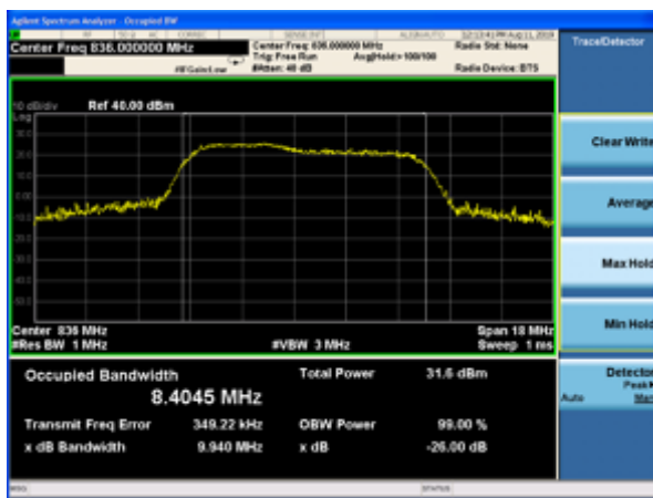
CA-5B 64QAM 5MHz+3MHz-Middle
