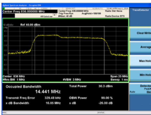
CA-5B 64QAM 5MHz+10MHz-Middle
