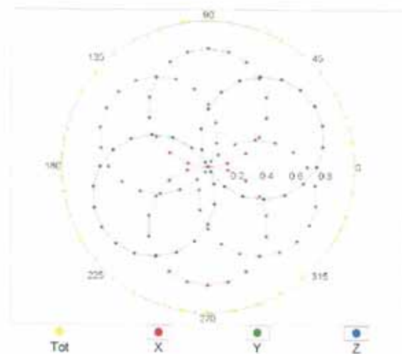
f=1800 MHz,R22
