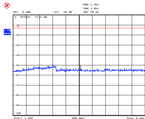
GSM 850 CH-High 1GHz ~ 9GHz
