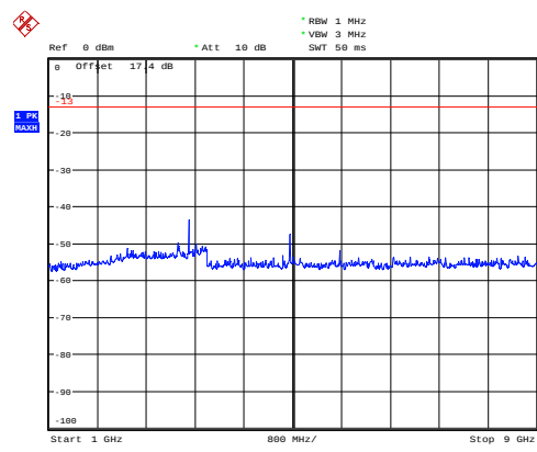
GSM 850 CH-Low 1GHz ~ 9GHz
