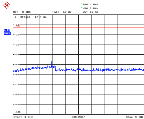
GSM 850 CH-Middle 1GHz ~ 9GHz
