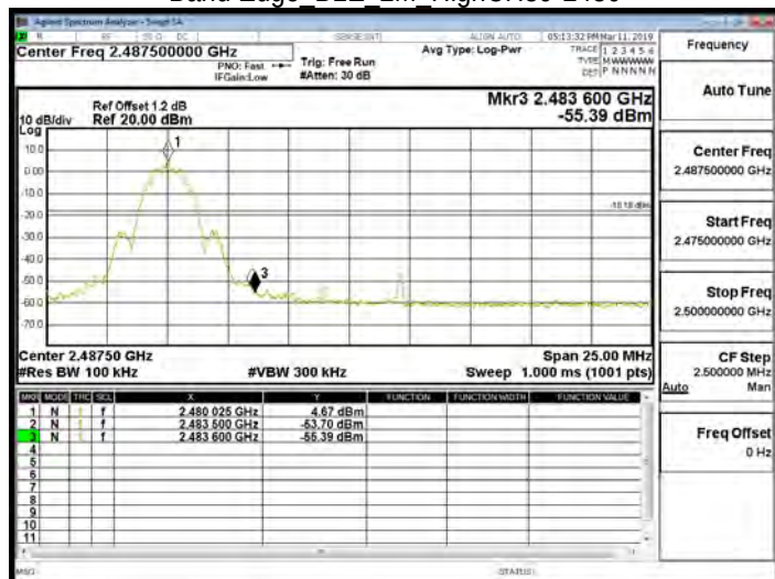
Band Edge BLE 2M HighCH39-2480
