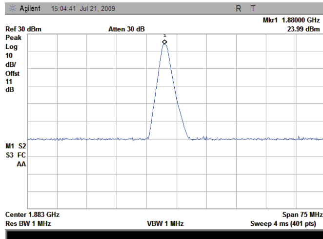
(Plot E: GSM 1900MHz Channel = 661)
