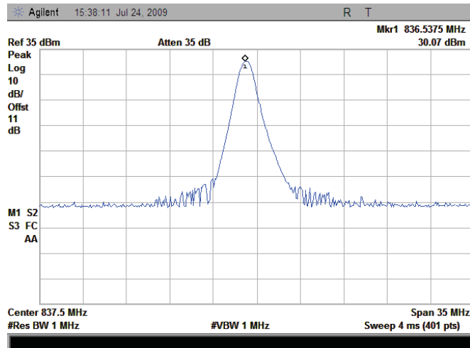
(Plot B: GSM 850MHz Channel = 190)
