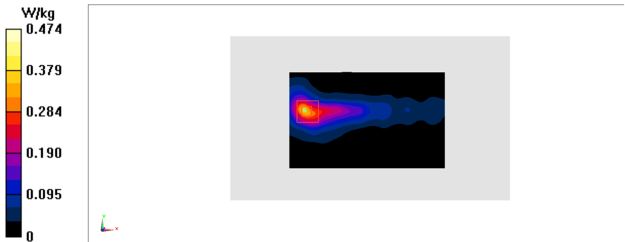
Fig.32 5GHz
