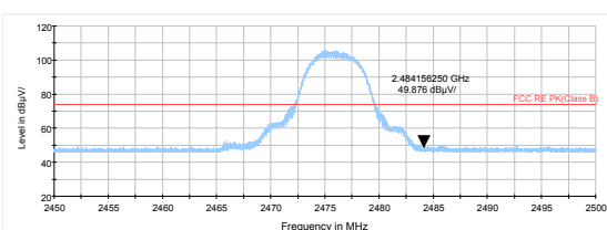
BT UHD 4M \pi/4 -DQPSK 2476MHz: Peak
