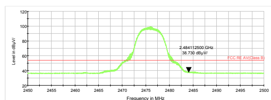
BT UHD 4M \pi/4 -DQPSK 2476MHz: Average
