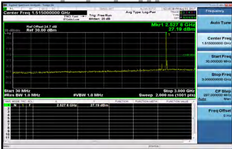
30MHz-3GHz_Band7_20MHz_QPSK_1_0_MidCH21100-2535
