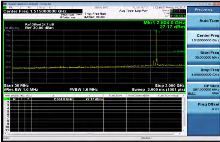
30MHz-3GHz_Band7_20MHz_QPSK_1_0_LowCH20850-2510
