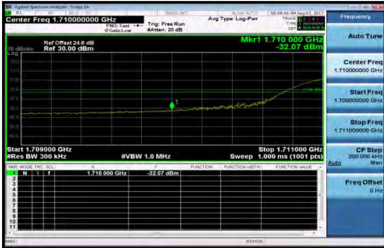
Band4_20MHz_QPSK_100_0_LowCH20050-1720
