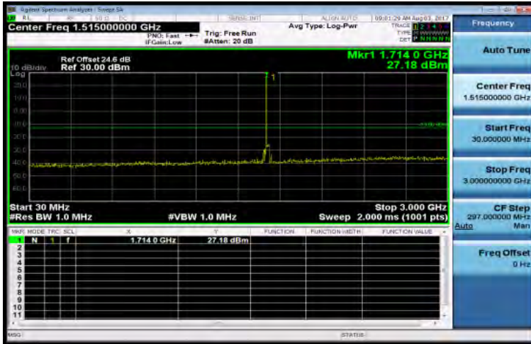
30MHz~3GHz_Band4_20MHz_QPSK_1_0_LowCH20050-1720
