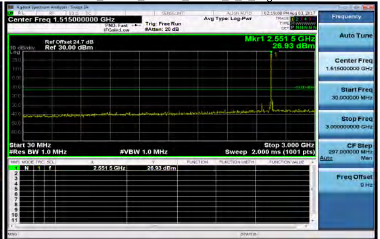
30MHz-3GHz_Band7_20MHz_QPSK_1_0_HighCH21350-2560
