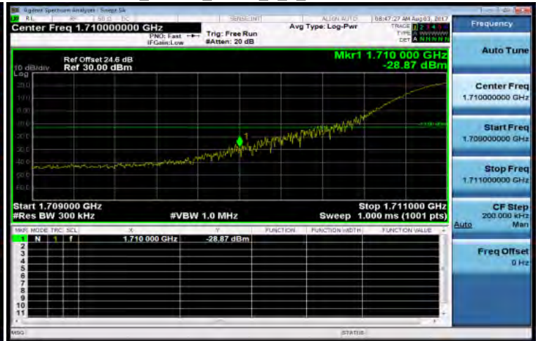
Band4_20MHz_QPSK_1_0_LowCH20050-1720
