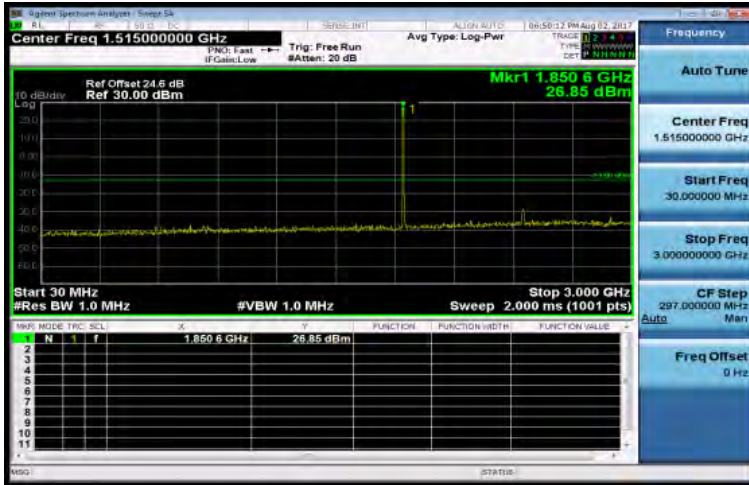
30MHz~3GHz_Band2_3MHz_QPSK_1_0_LowCH18615-1851.5
