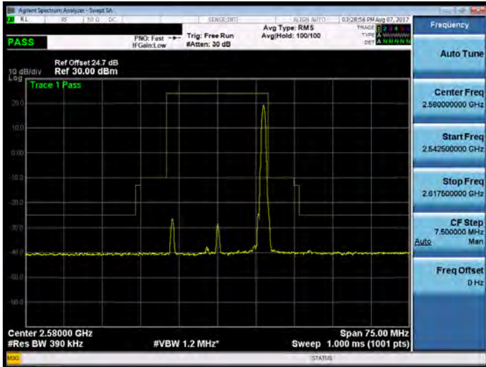
Band 38_20M_QPSK_LOW_RB100,0
