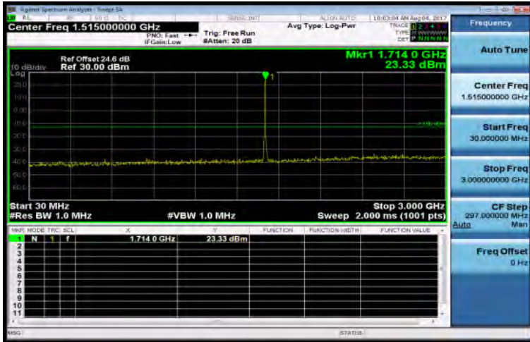
30MHz~3GHz_WCDMA_B4_LowCH1312-1712.4
