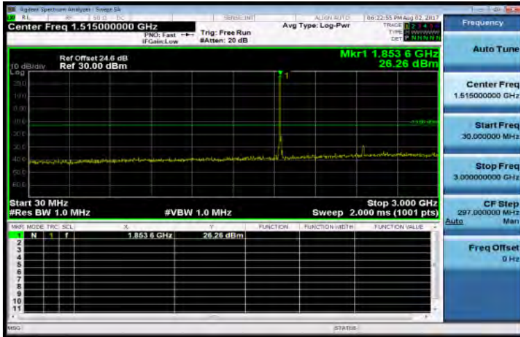
30MHz-3GHz_Band2_10MHz_QPSK_1_0_LowCH18650-1855
