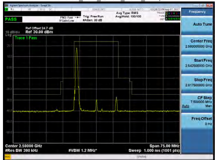
Band 38_20M_QPSK_LOW_RB1,0
