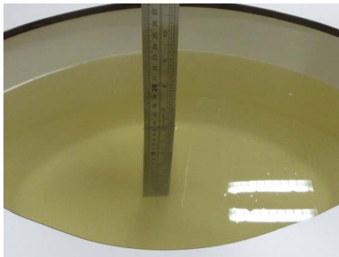
Body(835MHz)_15.6cm
