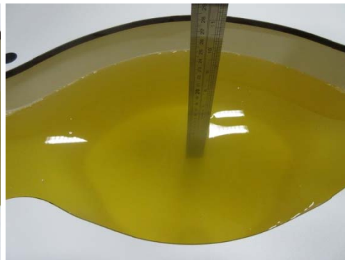
Body(1750MHz)_16.2cm
