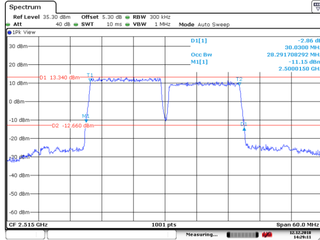
CA_7C_QPSK_75RB+75RB_20825+20975_PCC:75RB@0_SCC:75RB@0
