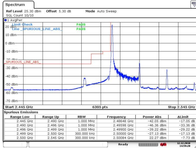
CA_7C_QPSK_75RB+75RB_20825+20975_PCC:1RB@0_SCC:0RB@0
