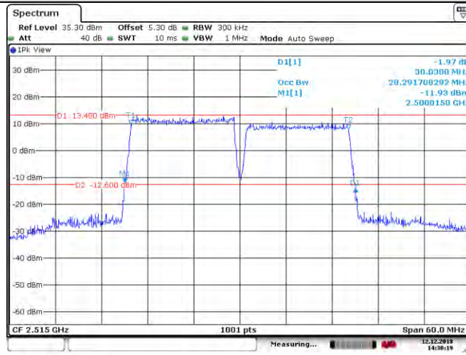
CA_7C_16QAM_75RB+75RB_20825+20975_PCC:75RB@0_SCC:75RB@0
