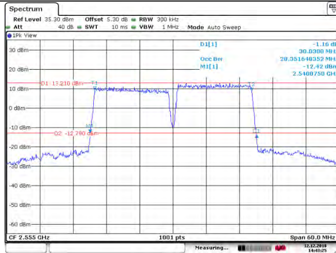
CA_7C_16QAM_75RB+75RB_20825+20975_PCC:75RB@0_SCC:75RB@0
