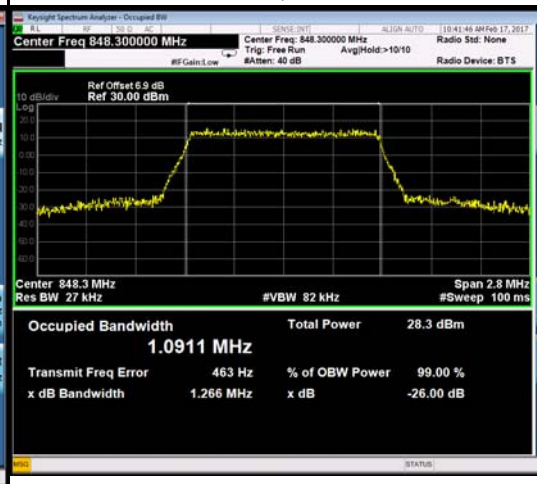
16QAM-20643
