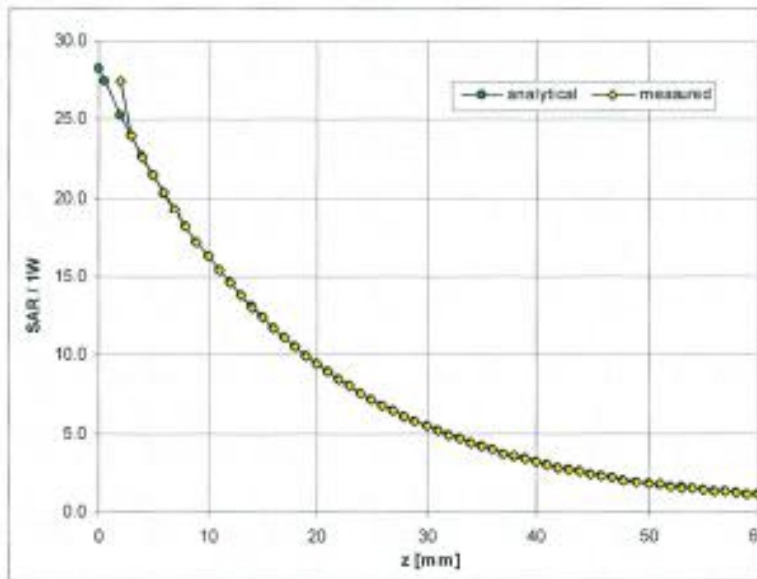
900MHz
