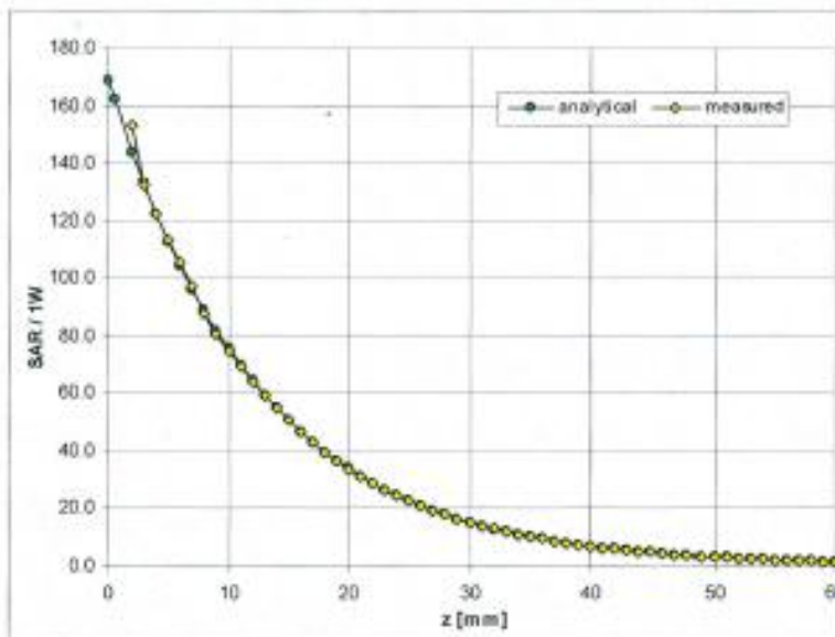
1900MHz
