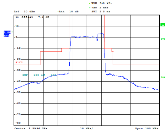
CA_41C 20MHz+5MHz QPSK RB=100#0+25#0 CH- Middle
