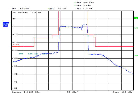
CA_41C 20MHz+5MHz QPSK RB=100#0+25#0 CH- High
