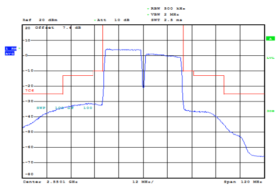
CA_7C 20MHz+20MHz QPSK RB=100#0+100#0 CH- High
