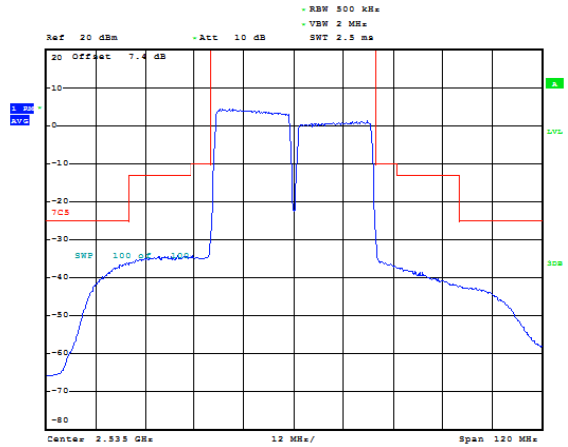
CA_7C 20MHz+20MHz QPSK RB=100#0+100#0 CH- Middle
