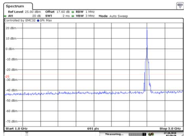
CA_38C 20MHz+20MHz CH- High 1GHz~3GHz
