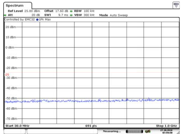
CA_38C 20MHz+20MHz CH- High 30MHz~1GHz
