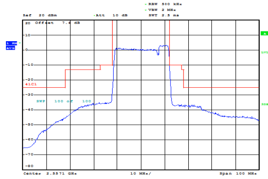
CA_41C 20MHz+5MHz QPSK RB=100#0+25#0 CH- Low
