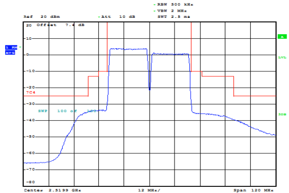
CA_7C 20MHz+20MHz QPSK RB=100#0+100#0 CH- Low
