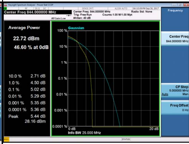
16QAM-26990
