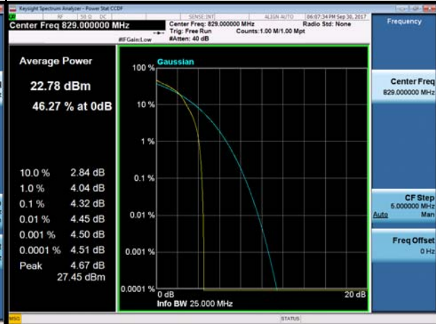
16QAM-26990
