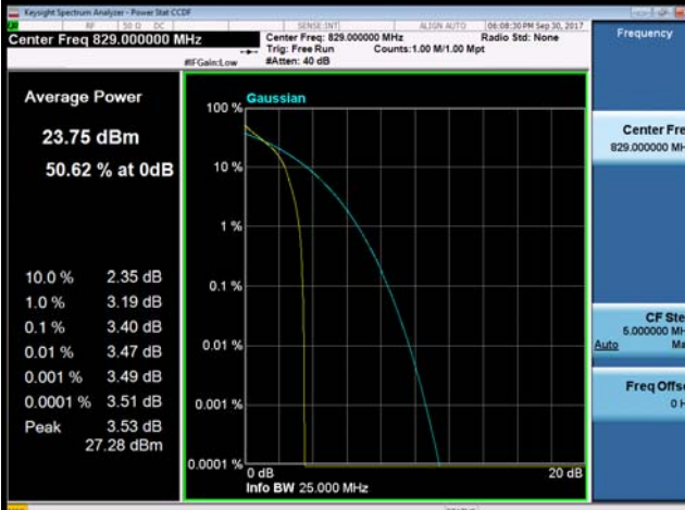
QPSK-26990
