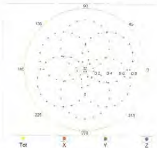
f=1800 MHz,R22
