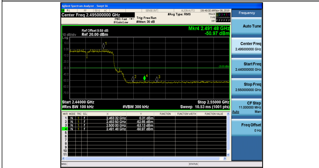
11N40MIMO_Ant2_High_2452
