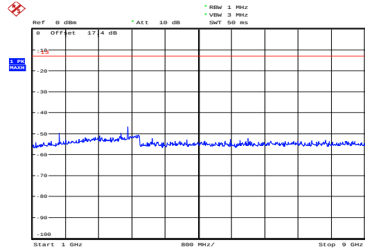
GSM 850 CH-Low 1GHz ~ 9GHz
