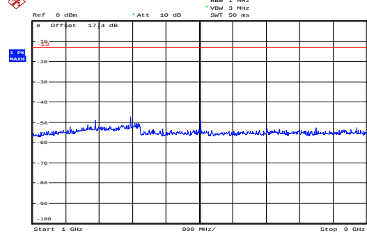
GSM 850 CH-Middle 1GHz ~ 9GHz
