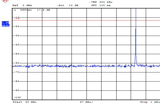
GSM 850 CH-Middle 30MHz ~ 1GHz
