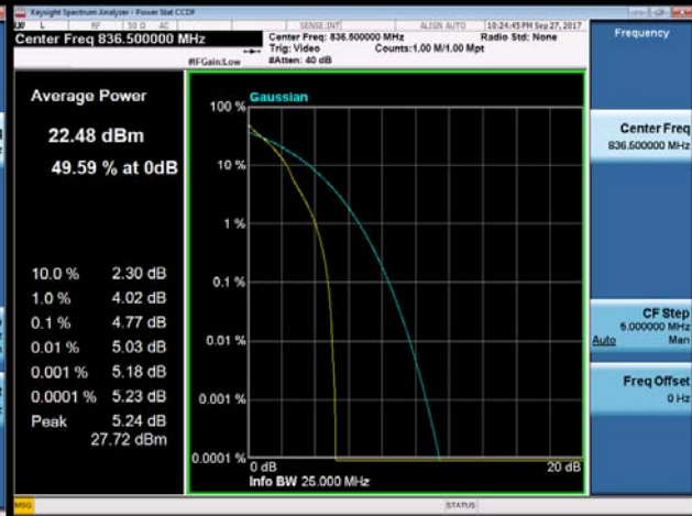
16QAM-26865
