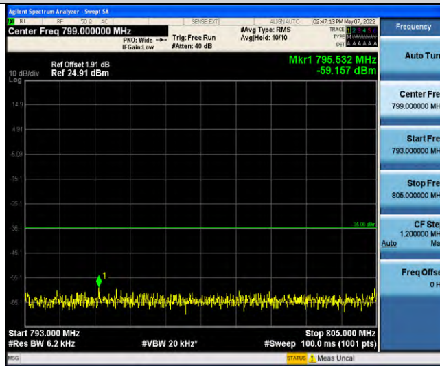
Band13-Stand-Alone-Na-N-QPSK-23182-1 @0-3.75kHz-793-805-793~805MHz @ -59.16dBm--35-PASS
