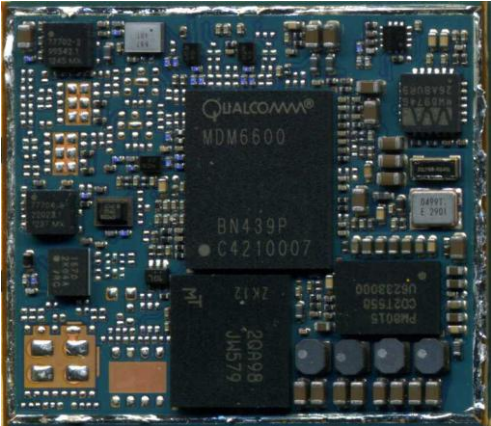
PVS8 Top side
