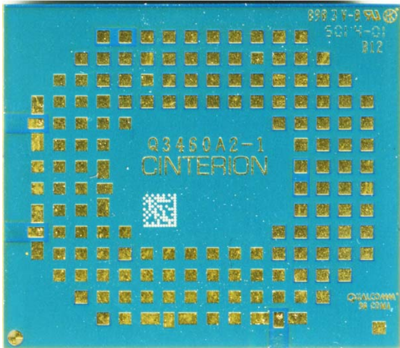
Bottom Side
