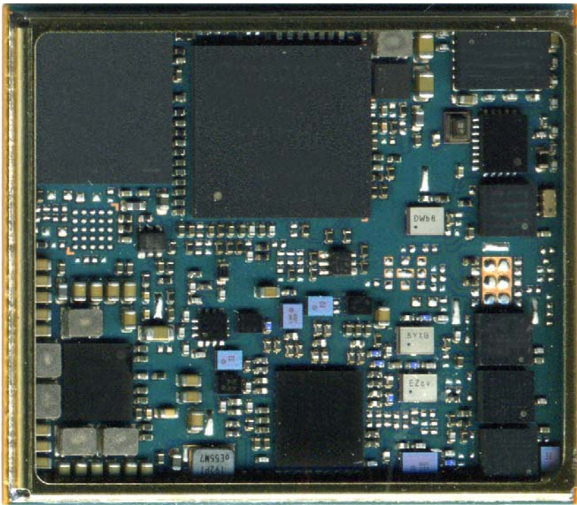
Top Side
