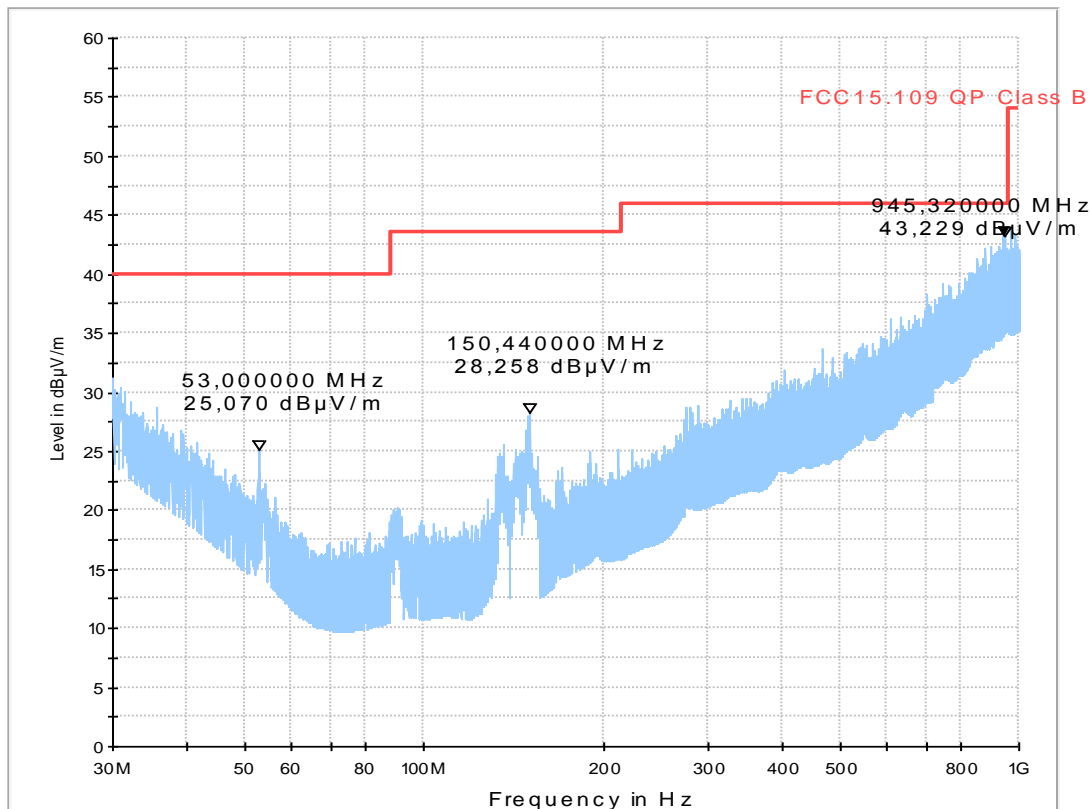
18_FCC15.109_Class B_hor+vert_kipp
