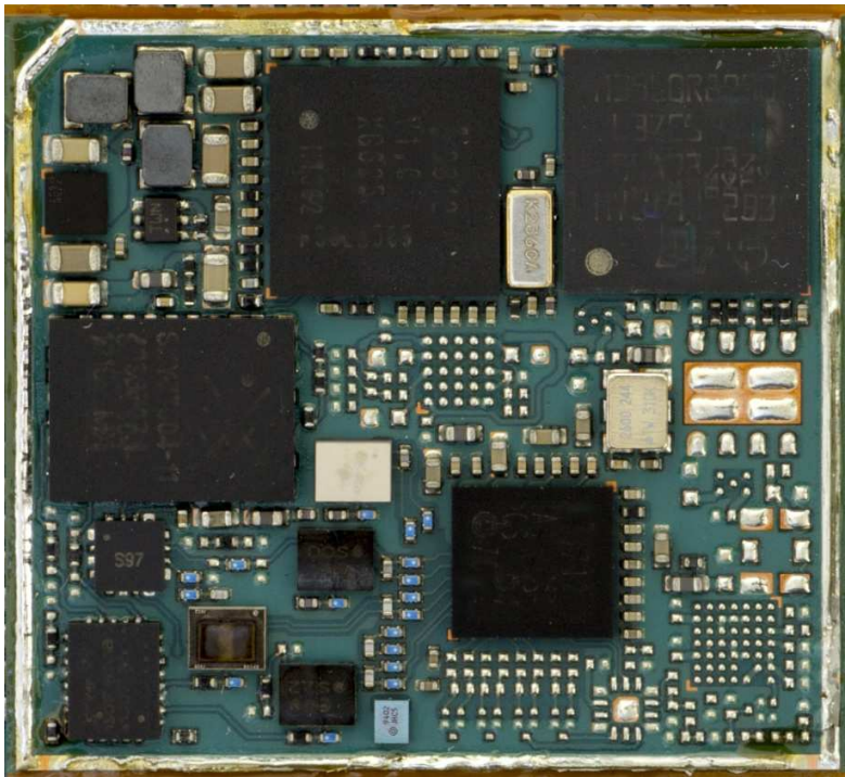
Top Side
