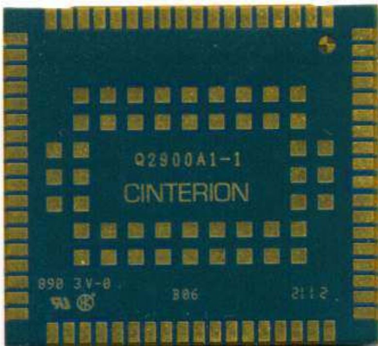
Bottom Side
