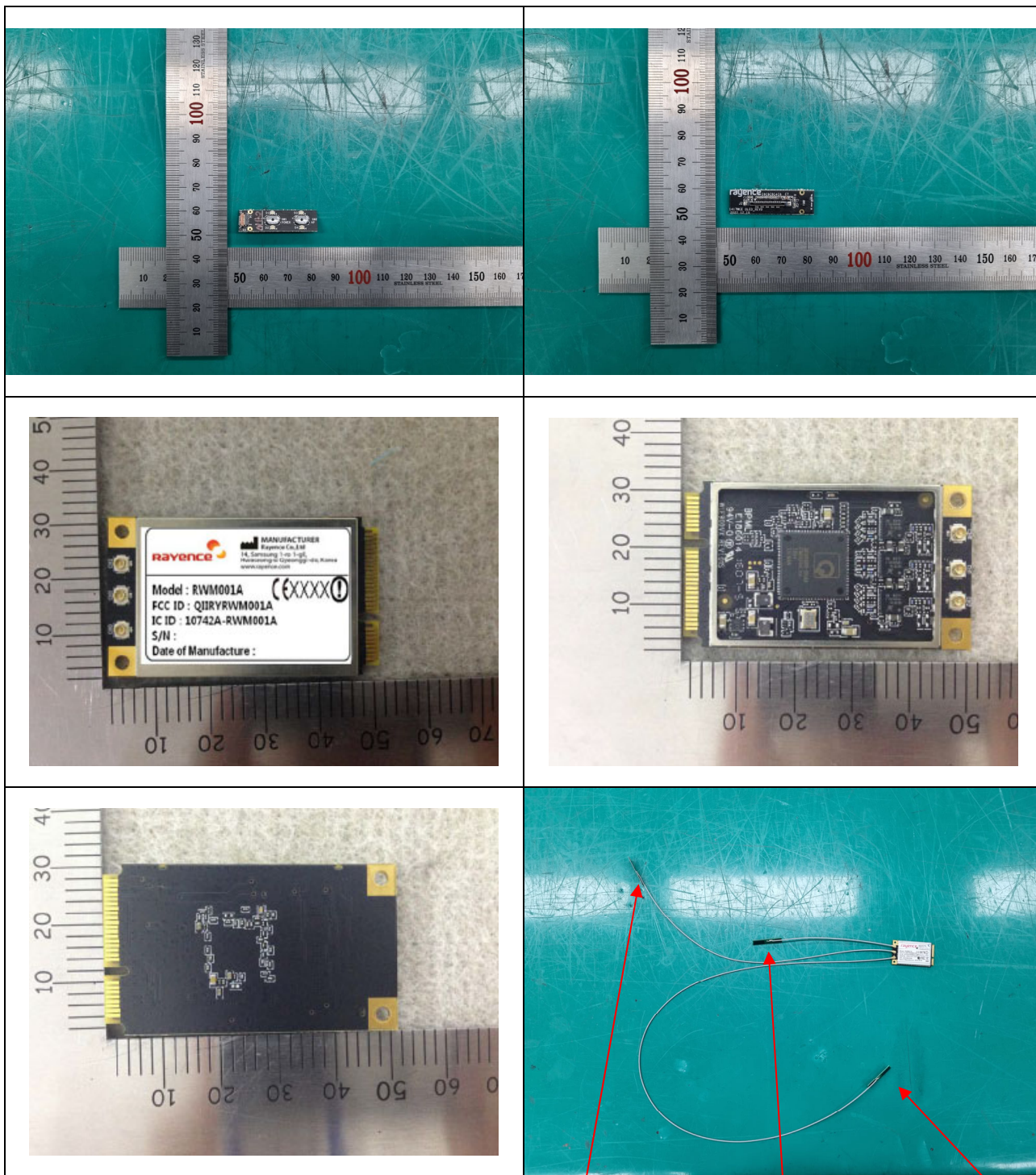
RAT011A Antenna
