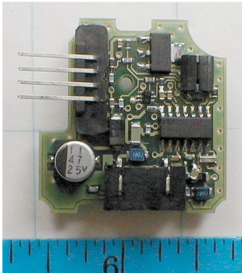
PCB Top
