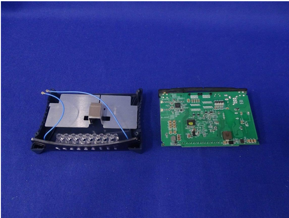
(8) EUT Photo
