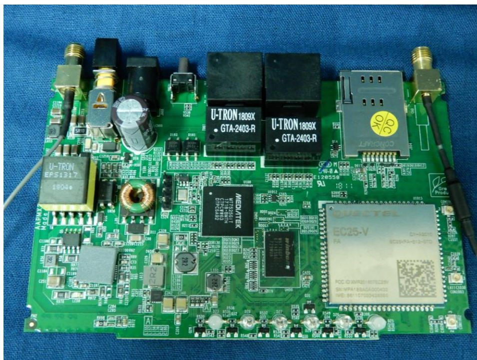
(14) EUT Photo
