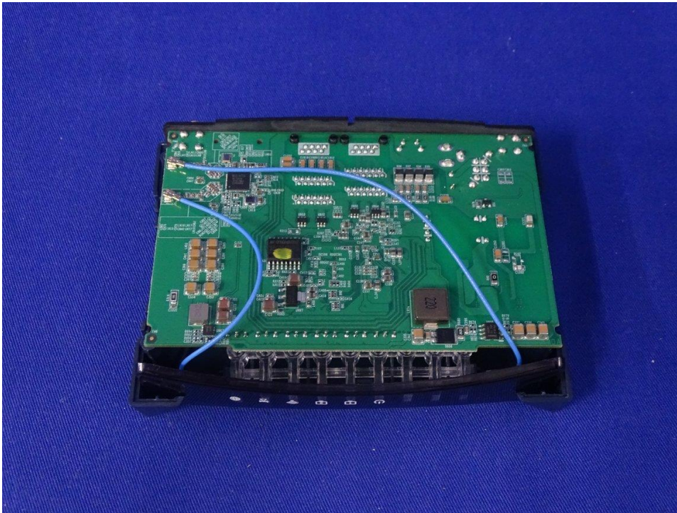
(8) EUT Photo
