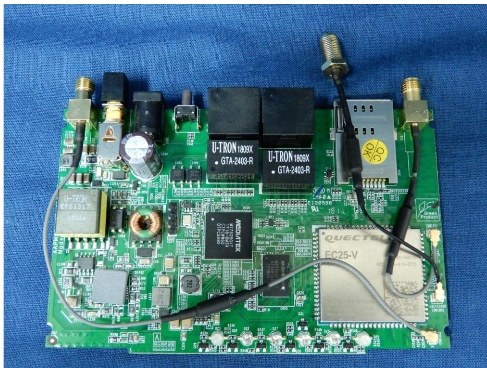
(14) EUT Photo
