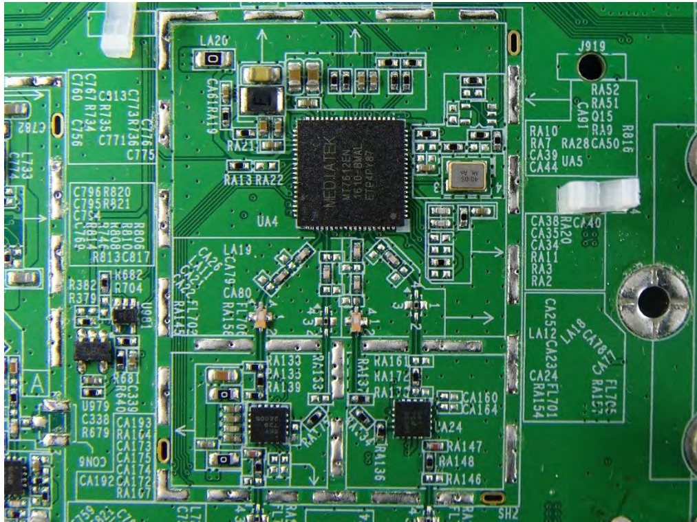
(21) EUT Photo_5GHz Module
