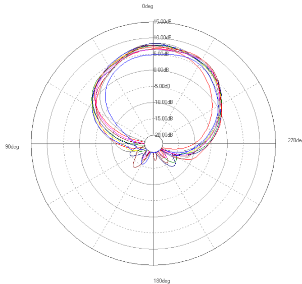
H-plane
