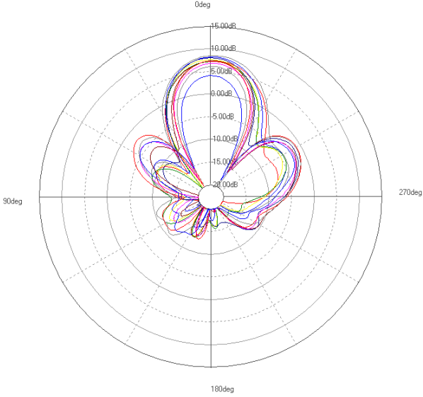
V-plane
