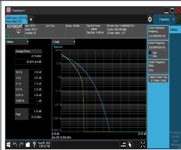
30MHz_QPSK_CH641666
