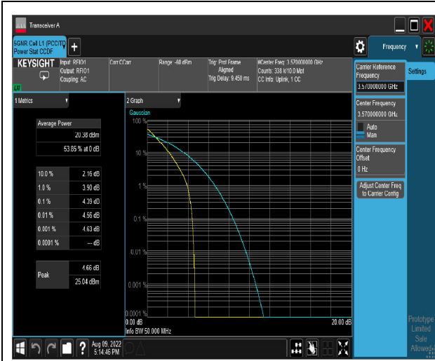
40MHz_PI/2 BPSK_CH638000
