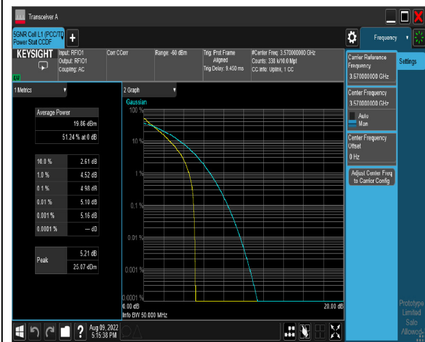
40MHz_QPSK_CH638000
