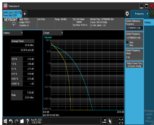
40MHz_PI/2 BPSK_CH645332
