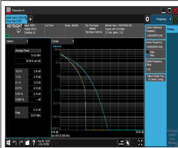
30MHz_QPSK_CH637668
