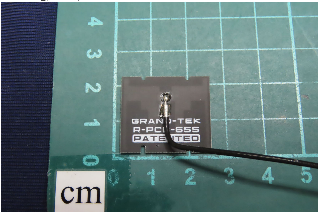
(20) EUT Photo_(Antenna)
