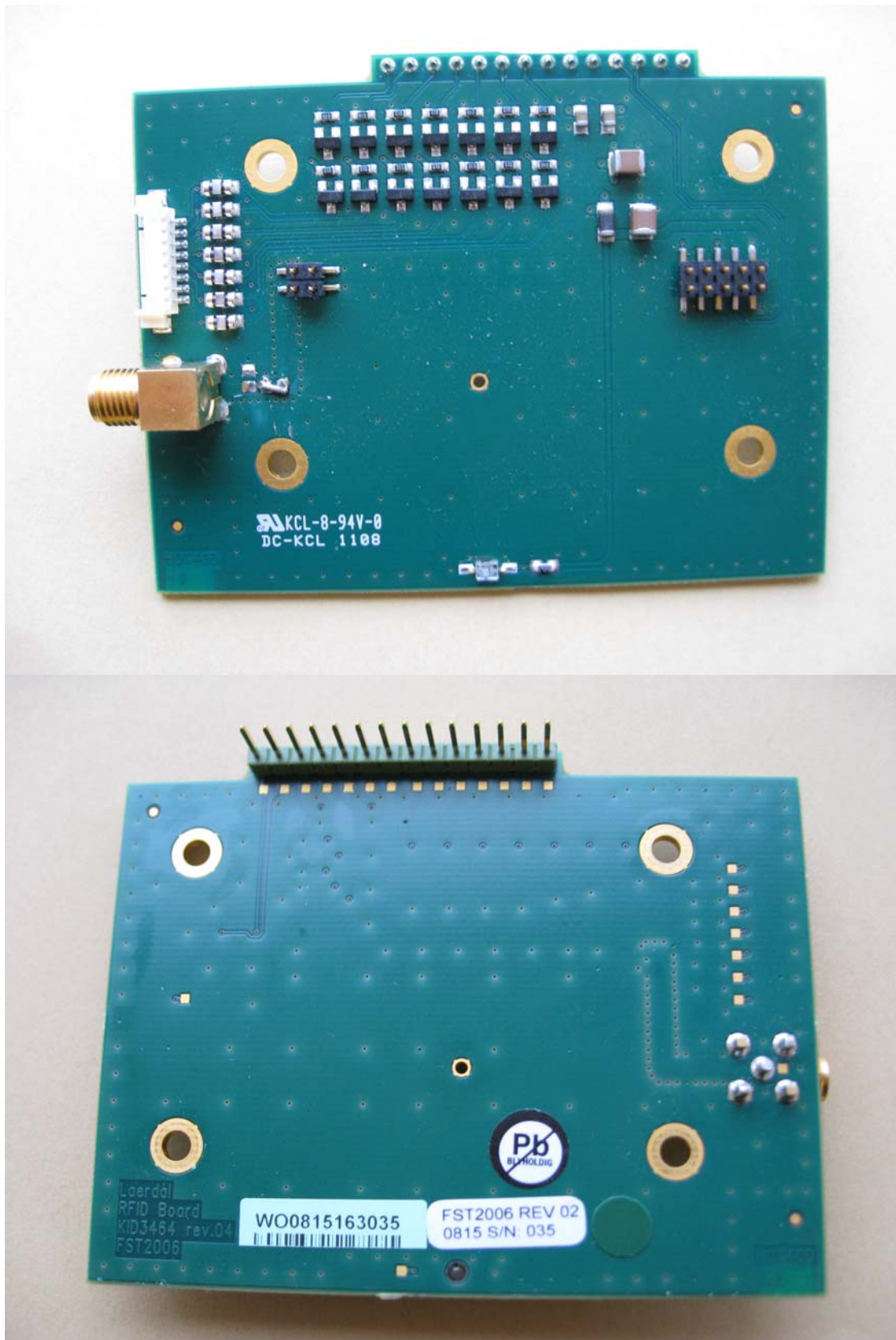
RFID Board FST2006
