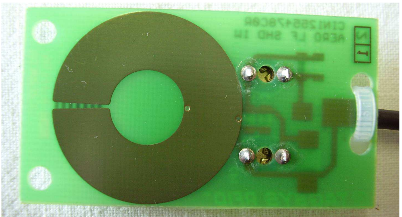
AERO-LF antenna
