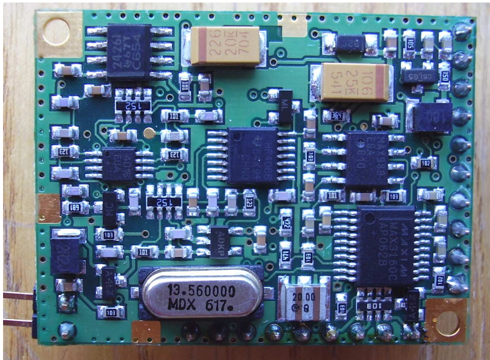
S002 module
