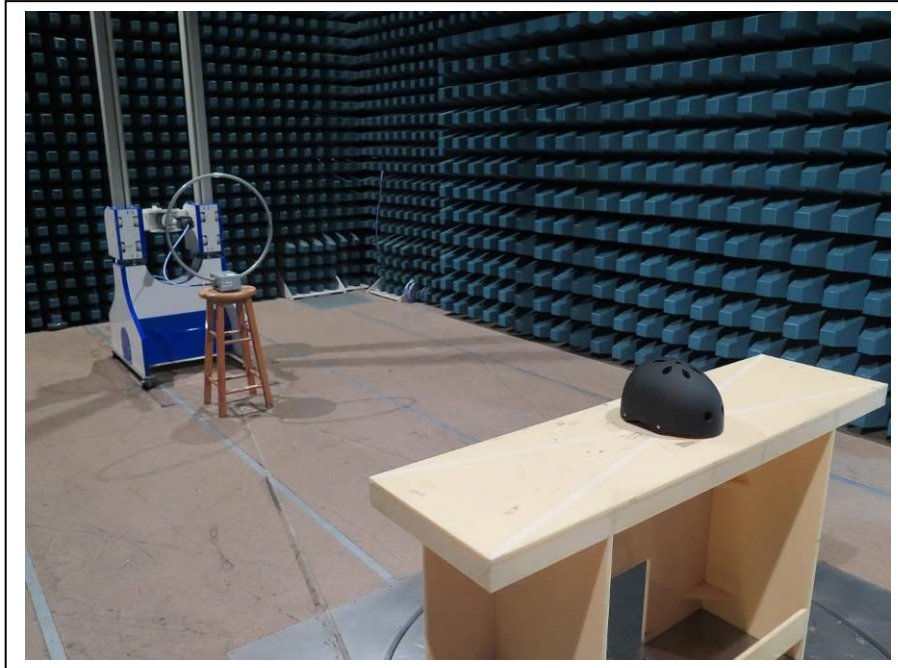
9kHz – 30MHz
