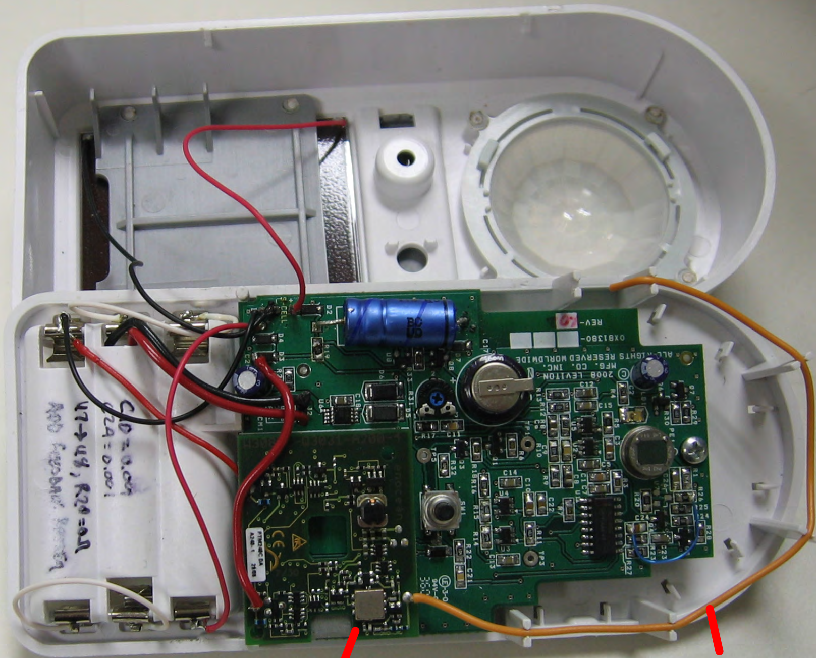
Antenna
