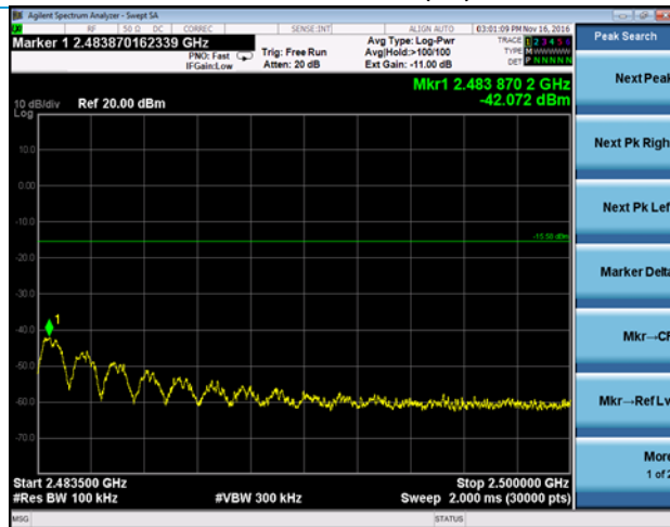
Upper band edge (26)
