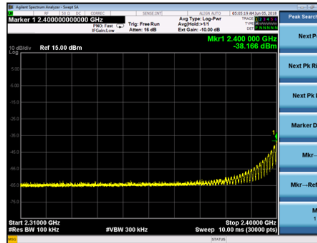
Lower Band Edge (CH 11)
