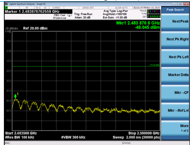
Upper Band Edge (CH 25)
