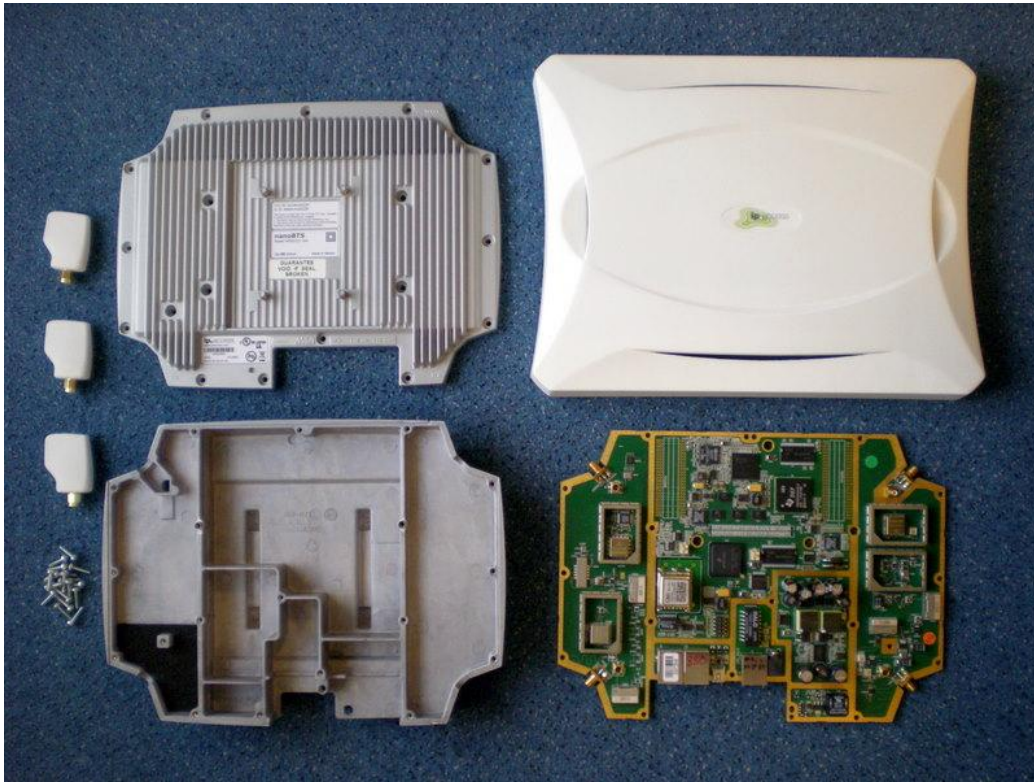
165D-Parts
