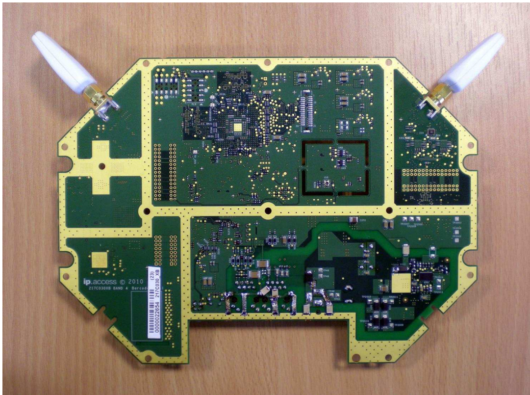
217C - PCB(Bottom)
