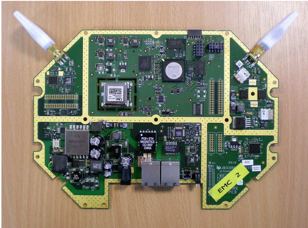
217C - PCB(Top)
