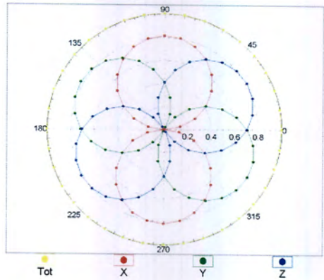
f=1800 MHz,R22
