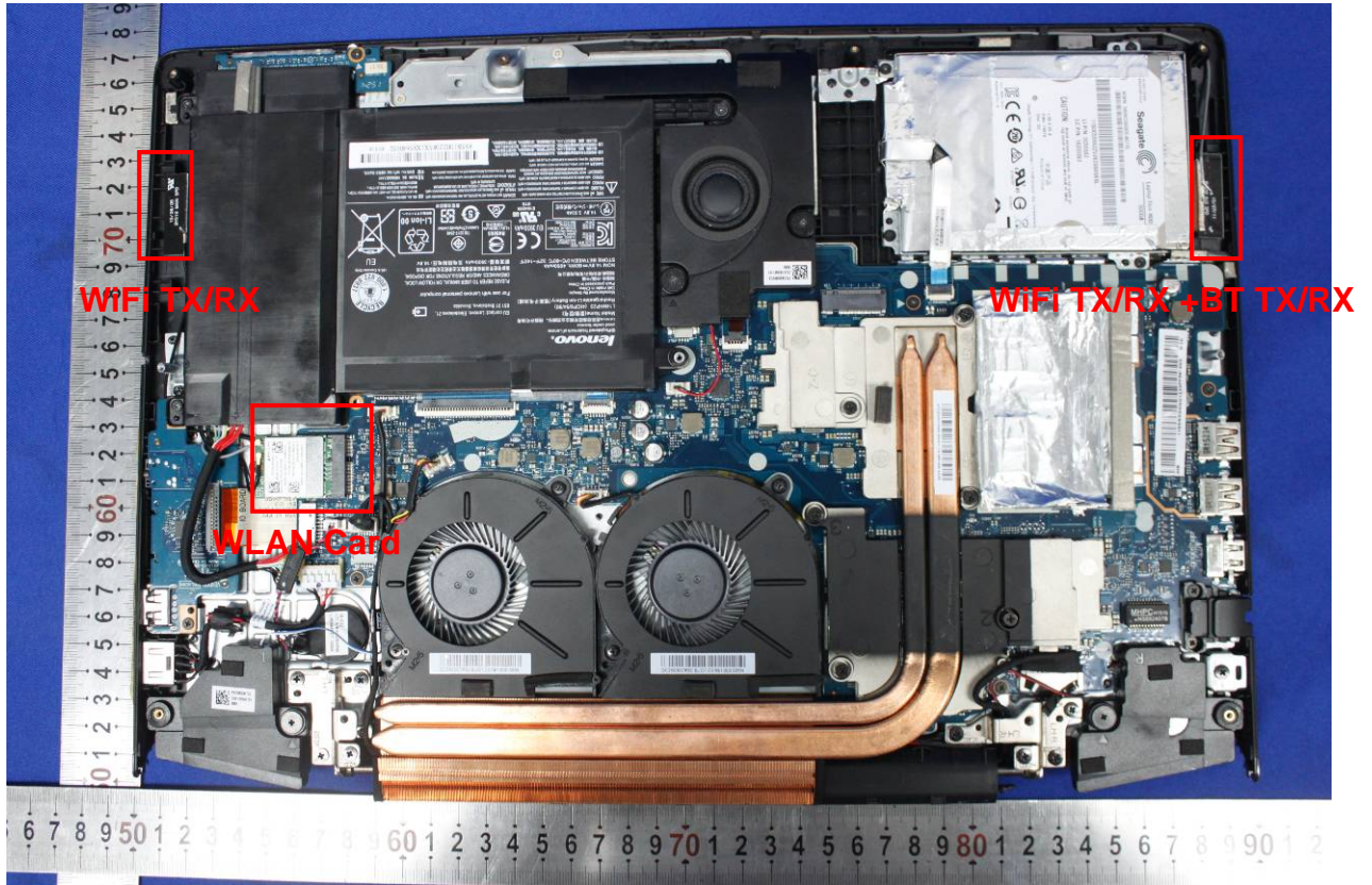
(2) EUT photo
