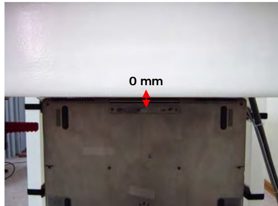
Fig.6 EUT Edge 4 mode to flat phantom
