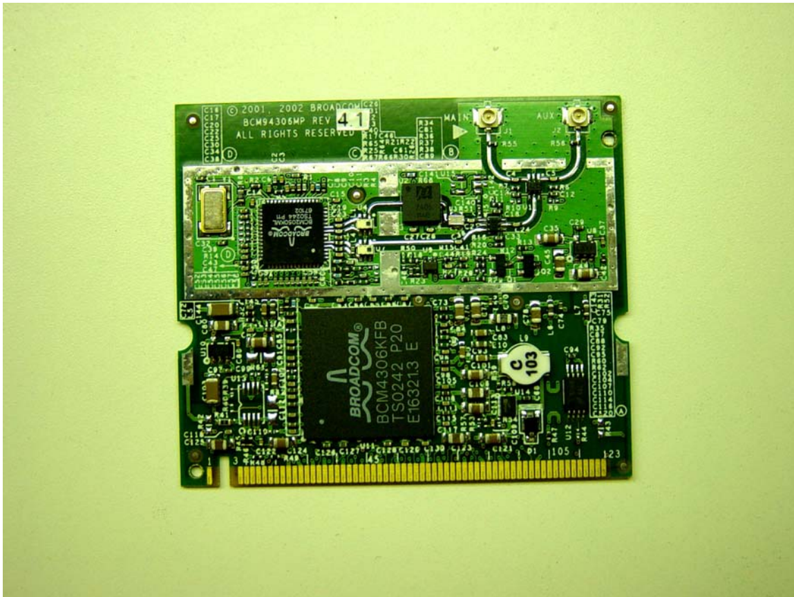
Photo 1. EUT top
