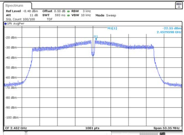
802.11n_HT40 / 2 452 MHz
